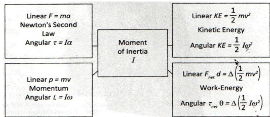
Gambar 3.6 Hubungan Momen Inertia Dengan Gaya, Momentum, KE, dan WE
